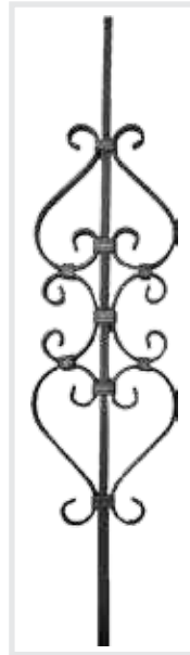
▶M-74 H.800xL.170mm ∅12
