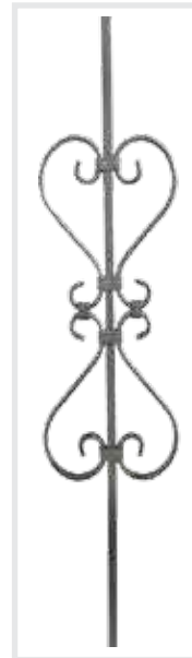
▶M-59 H.800xL.170mm ∅12
